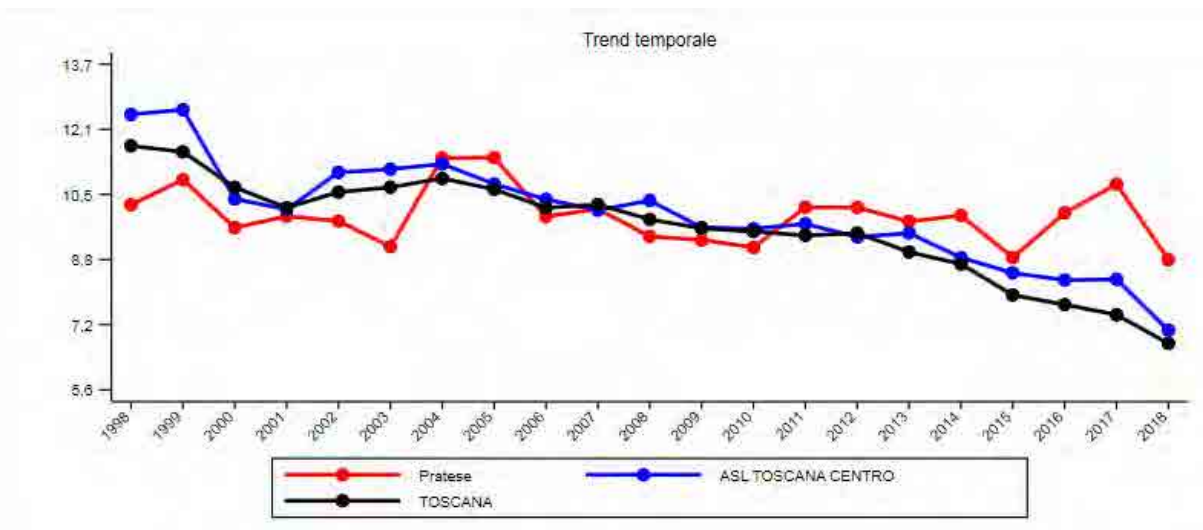
Figura 31. Andamento temporale del tasso di ospedalizzazione per IVG in donne in età fertile (14-49anni) nel 2018.
